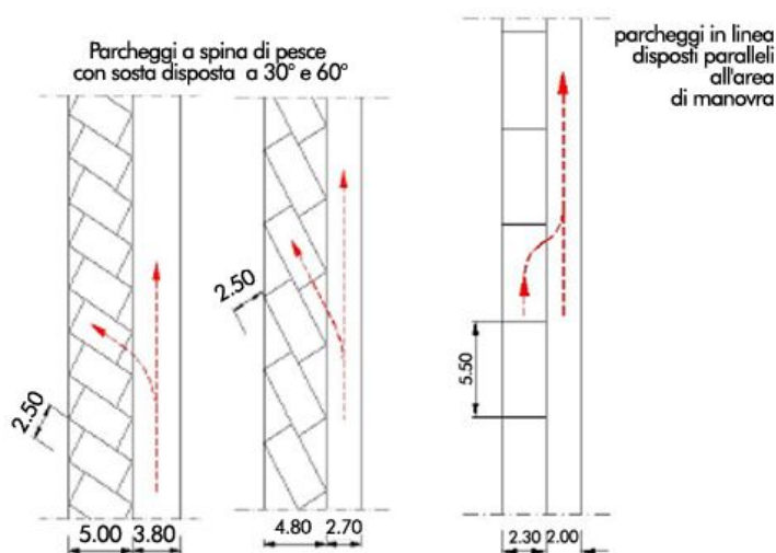
Fig. n°3 – Criteri di realizzazione dei parcheggi
