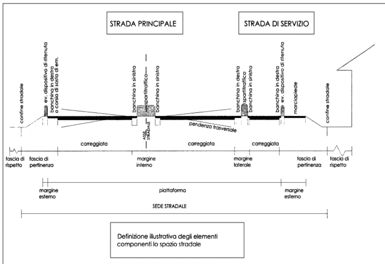
Figura 92.1 Elementi costitutivi dello spazio stradale (D.M. 5 novembre 2001) Sezione tipo
