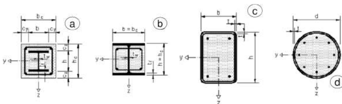
Figura 66.1 Tipi di sezioni per colonne composte adottate nel progetto
