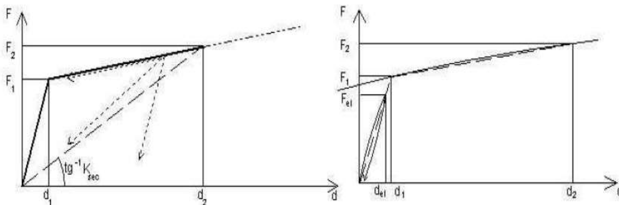
Figura 67.1 Diagrammi forza-spostamento per dispositivi non lineari
